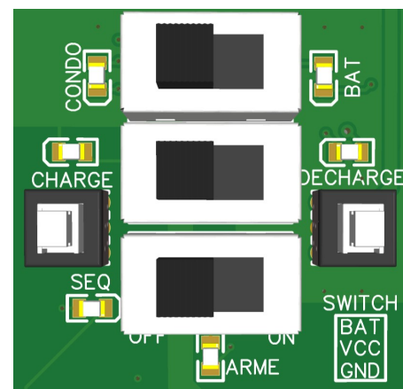
FIGURE 1.11 – Zoom sur l'interface de la carte principale du système d'allumage
