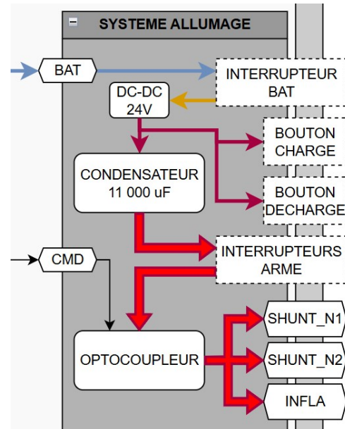
FIGURE 1.5 – Zoom sur le synopsis de la ligne de mise à feu (ref. annexe ??)
